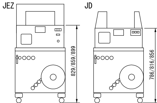
機械テーブル高さ寸法
